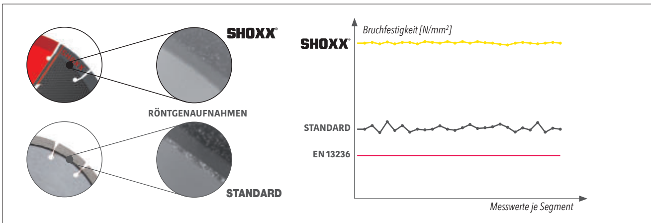
Porentiefe Verschweißung der SHOXX -Segmente
