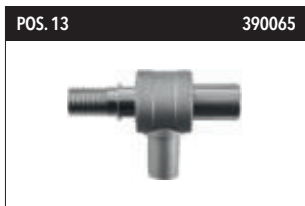
POS. 13 390065 KBZ 500 Absaugrotor für Trockenbohrungen Präzise Ganzmetallausführung zur effektiven Staubabsaugung beim Trockenbohren. Erhöht Schnittgeschwindigkeit und Lebensdauer der Bohrkronen, verhindert „Klemmer“. Geeignet für alle 1 1/4" Bohrkronen. Verwendbar mit allen handelsüblichen Industriesaugern.
