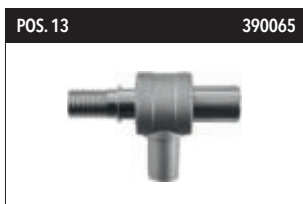
POS. 13 390065 KBZ 500 Afzuigrotor voor droge boringen Nauwkeurige volledig metalen uitvoering voor een effectieve stofafzuiging tijdens droog bo- ren, verhoogt de snij snelheid en levensduur van de boor- kronen, voorkomt vastklem- men. Geschikt voor alle 1 1/4" boorkronen. Te gebruiken met alle commercieel verkrijgbare industriestofzuigers.
