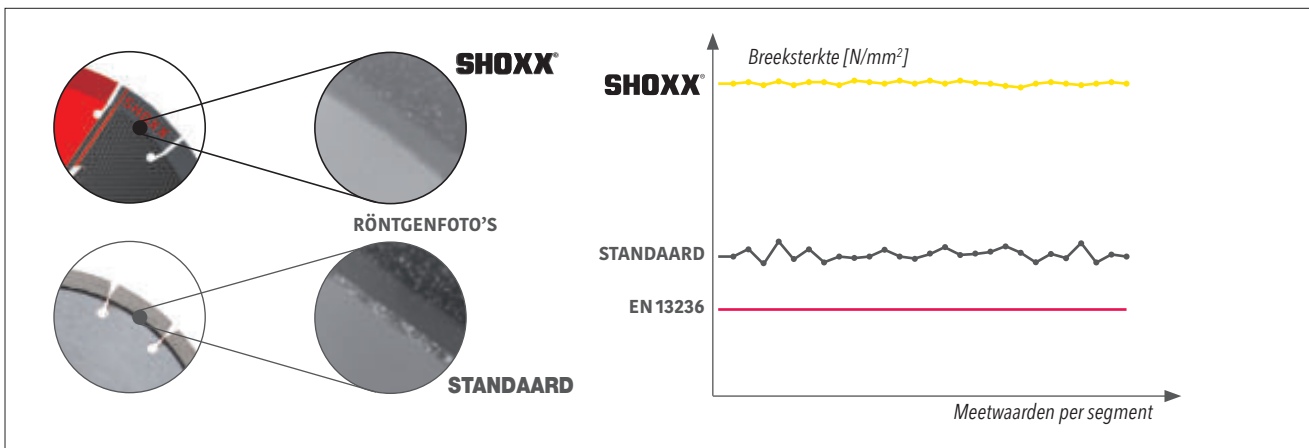
Poriëndiepe laswerk van SHOXX -segmenten
