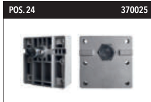
POS. 24 370025 KBZ 390 Montageplaat 6-gats RAPID LOCK Snelspaninrichting voor stationaire kernboormachine BMS 220 (390048).
