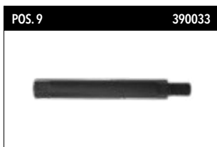
POS. 9 390033 KBZ 750 Prolongador para corona 300mm 1 1/4"
