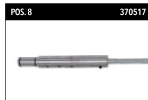
POS. 8 370517 KBZ 410 Guías de centrado para trabajar a mano alzada para coronas de longitudes 350-450 mm (aptas para motor de perforación BMF 200), conector
